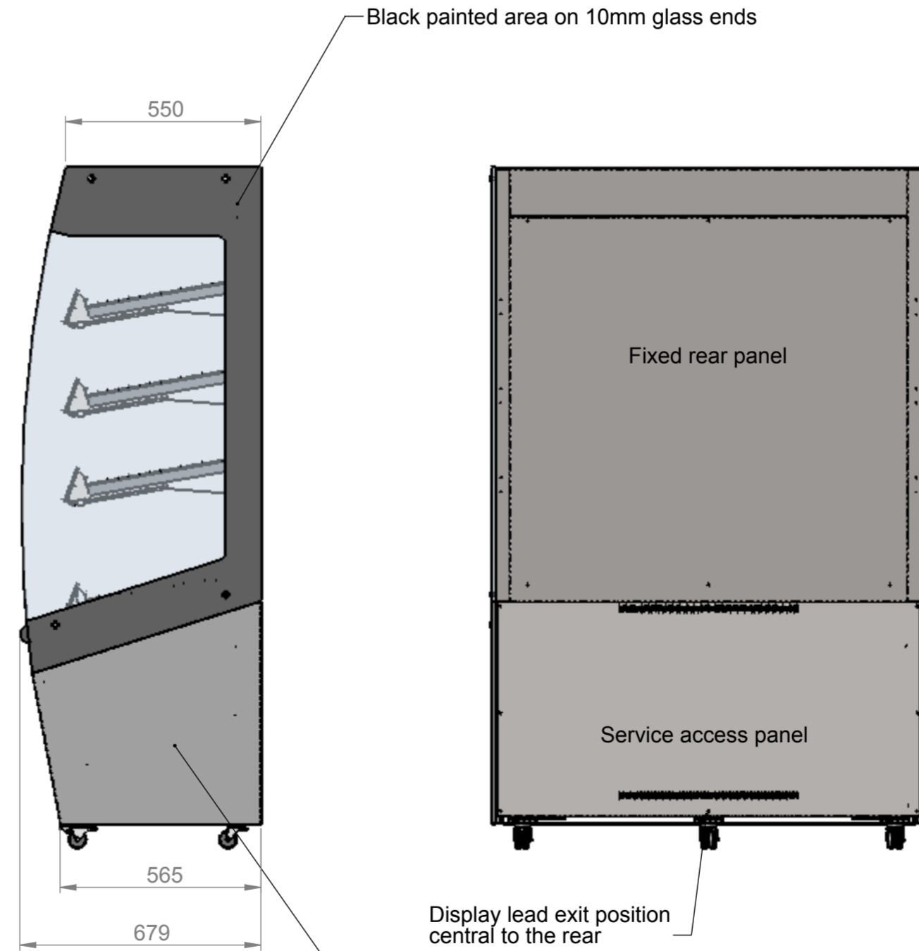
End elevation
